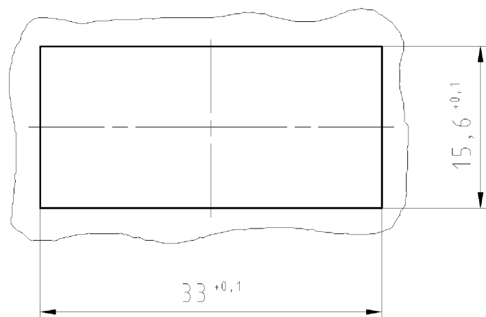
Blechausschnitt / sheet cutout t= 0,5-1,5 mm
