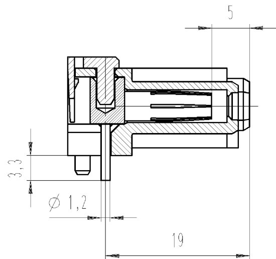
Schnitt A-A cross section
