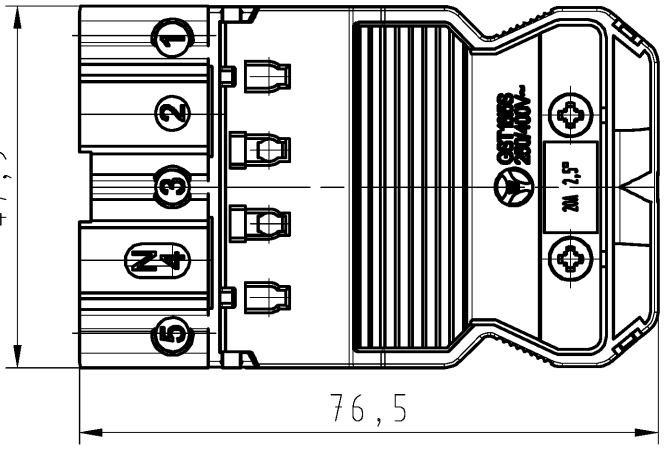
Darstellung im montierten Zustand view in assembled state
