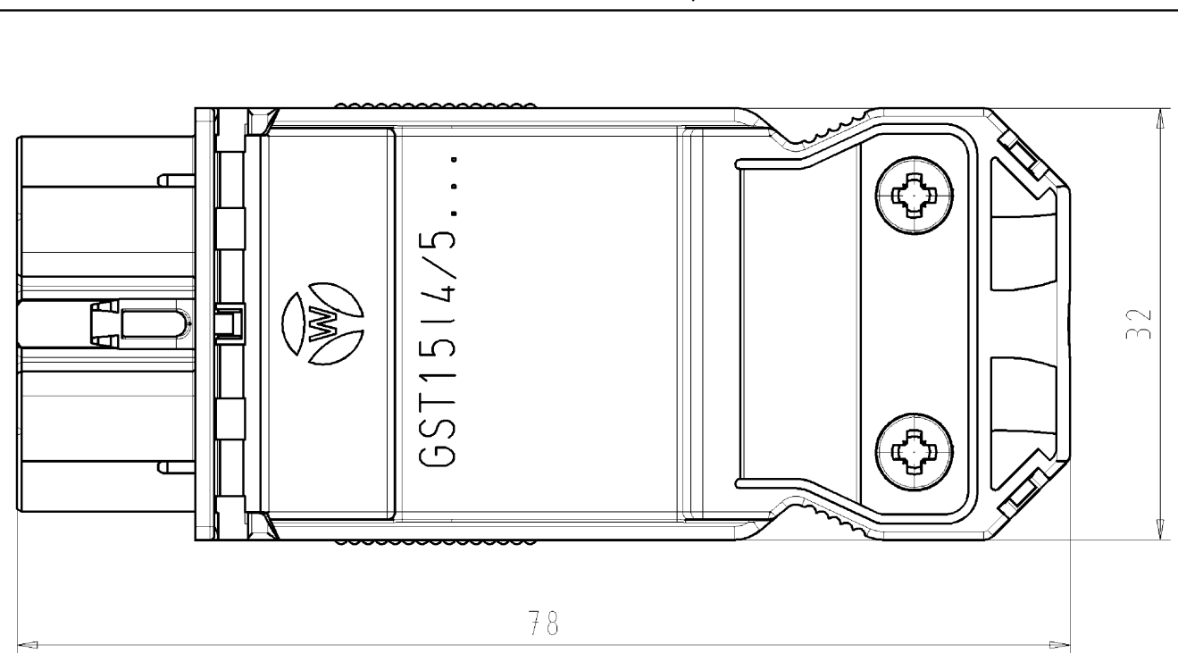
Ansicht im montierten Zustand / view in assembled state
