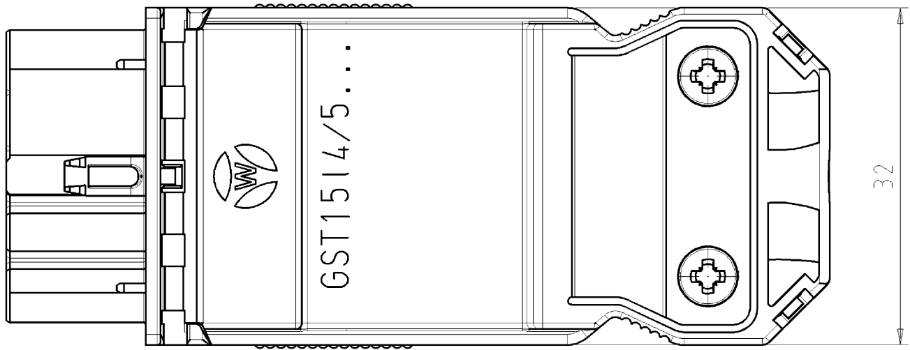
Ansicht im montierten Zustand / view in assembled state
