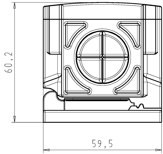
Ansicht in Pfeilrichtung "X" ohne Deckel gezeichnet view in arrow direction "X" drawn without cover
