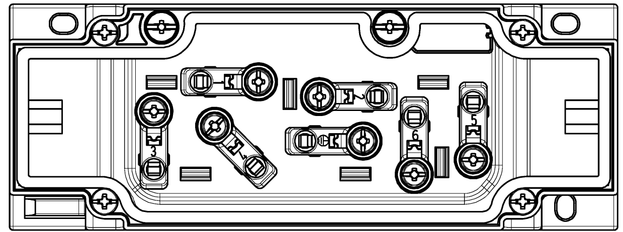
Ansicht in Pfeilrichtung "X" ohne Deckel gezeichnet view in arrow direction "X" drawn without cover
