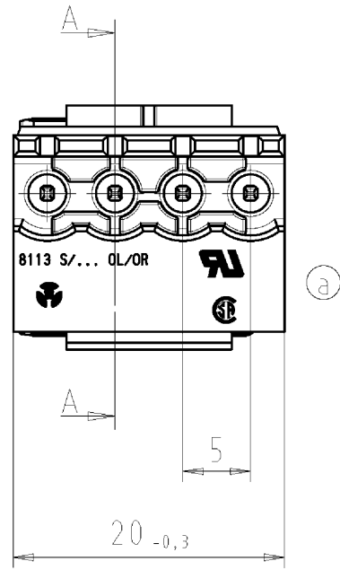
Ansicht von Hinten back view M5:1
