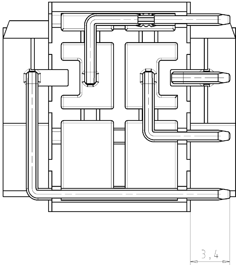
Ansicht von Hinten back view M5:1
