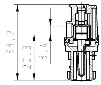
Schnitt A-A section A-A
