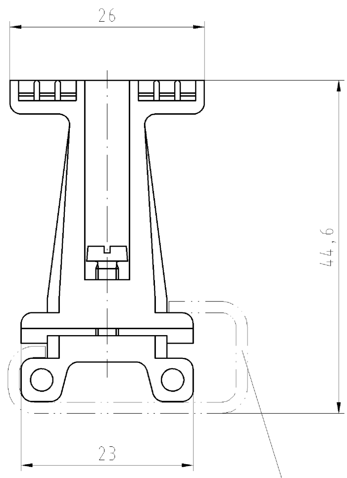
G-Schiene EN 60715 - G32 g-rail EN 60715 - G32
