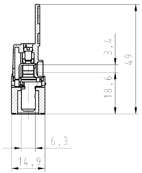
Schnitt A-A section A-A
