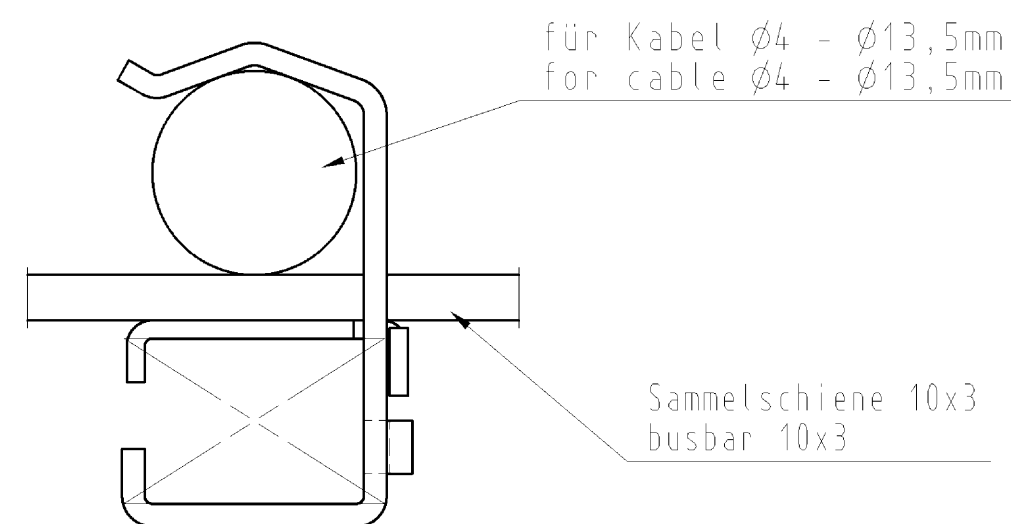
montierter Zustand/mounted state M 2:1
