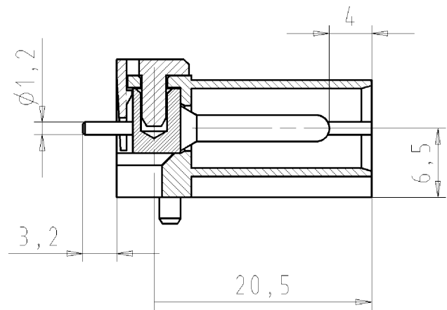
Schnitt/cross section C-C
