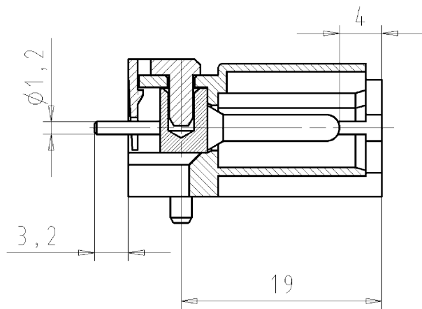
Schnitt/cross section A-A
