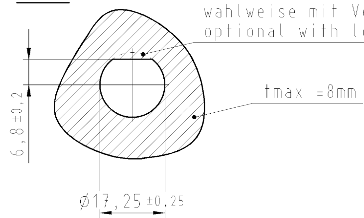
Gehäuseausschnitt cut out
