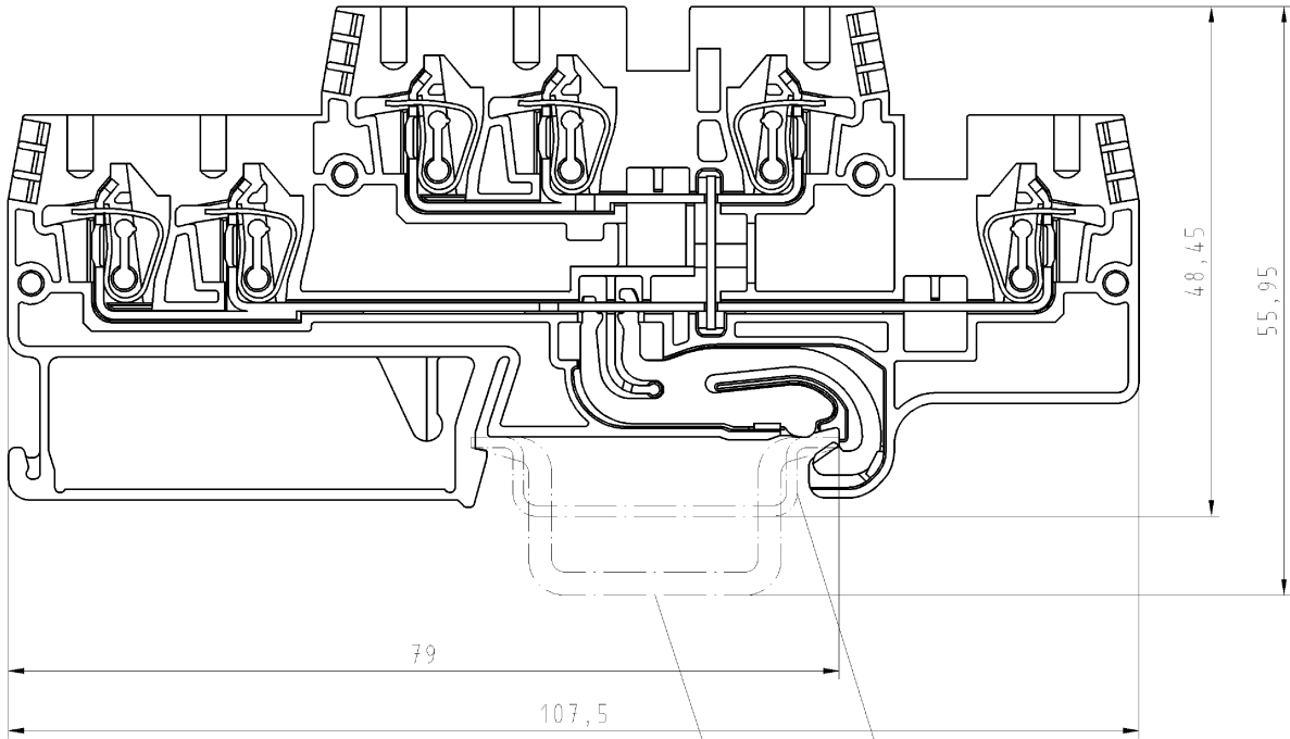
Hutschiene EN 60715-35x7,5 mounting rail EN 60715-35x7,5
