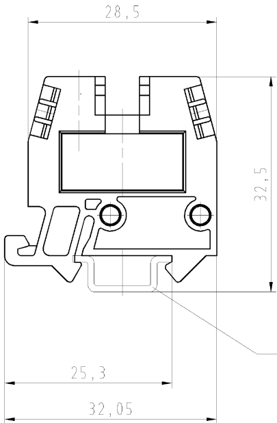
Hutschiene EN 60715-15x5,5 mountail-rail EN 60715-15x5,5
