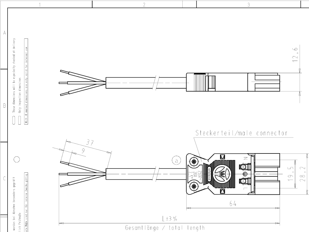
Kabel/cable H05VV-F3G2,5 Farbe/colour: siehe Tabelle/see table
