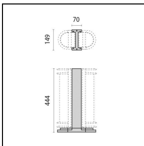
000445 Poteau 45 444 mm ■ GR-94 / Gris métallisé
