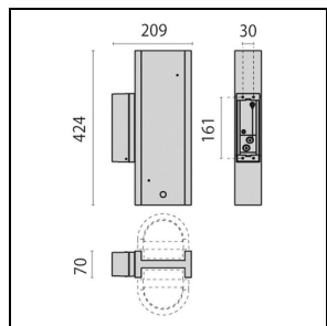
000441 Console 45 ■ GR-94 / Gris métallisé
