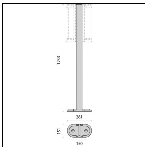
000453 Poteau 45 1233 mm ■ GR-94 / Gris métallisé
