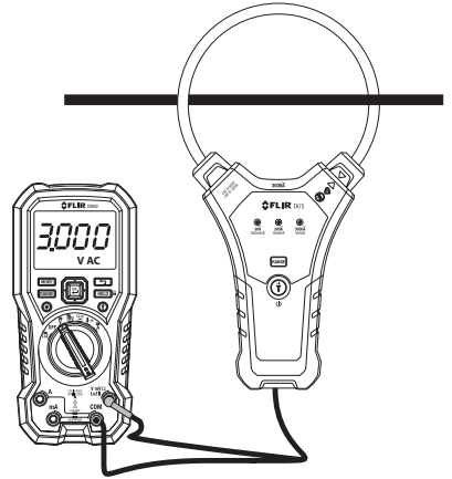
Fig. 5-1 Raccordement au DMM
