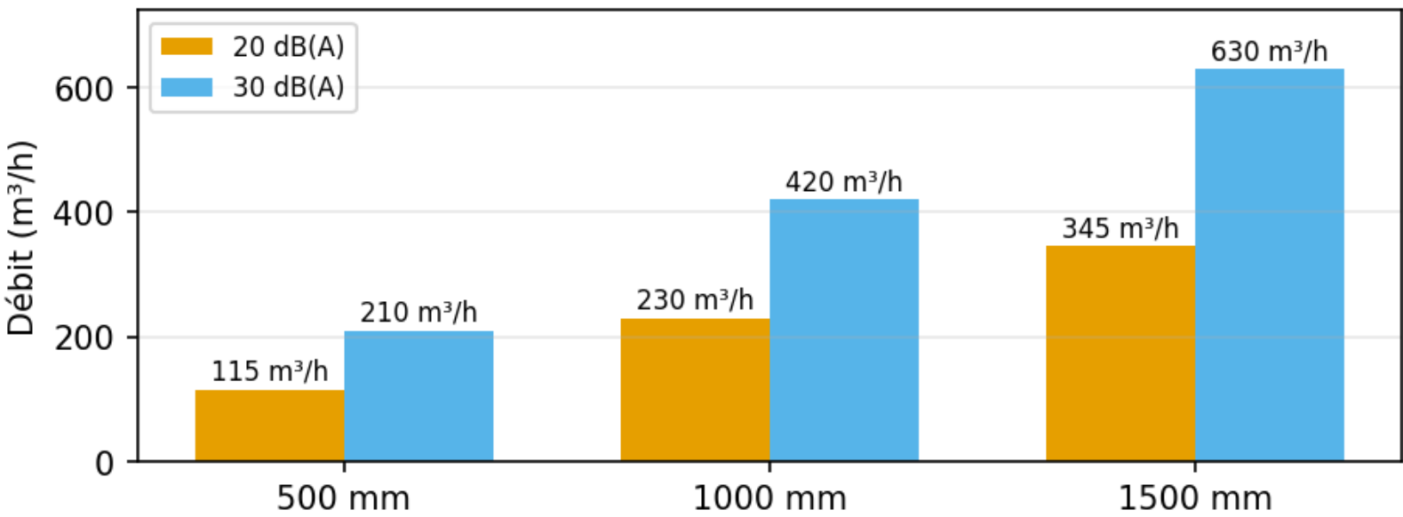
Débit par longueur — C2020 20
