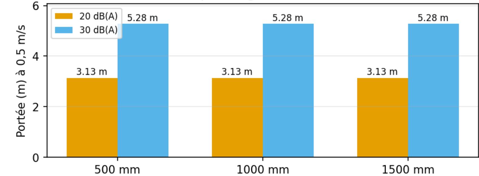
Portée par longueur — C2020 20
