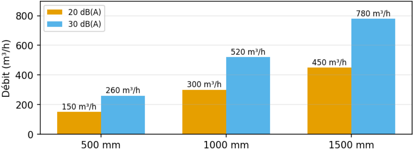
Débit par longueur — C2020 25
