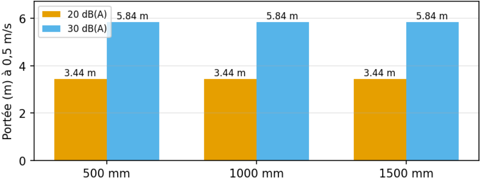
Portée par longueur — C2020 25
