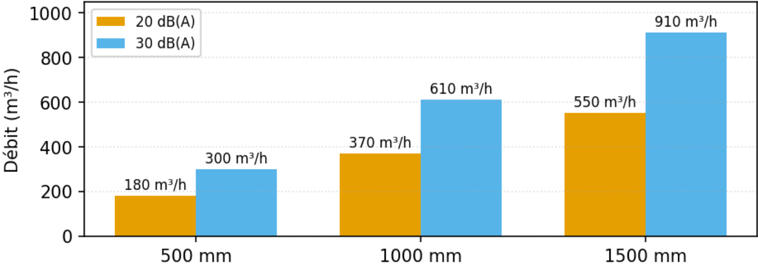
Débit par longueur — C2020 30
