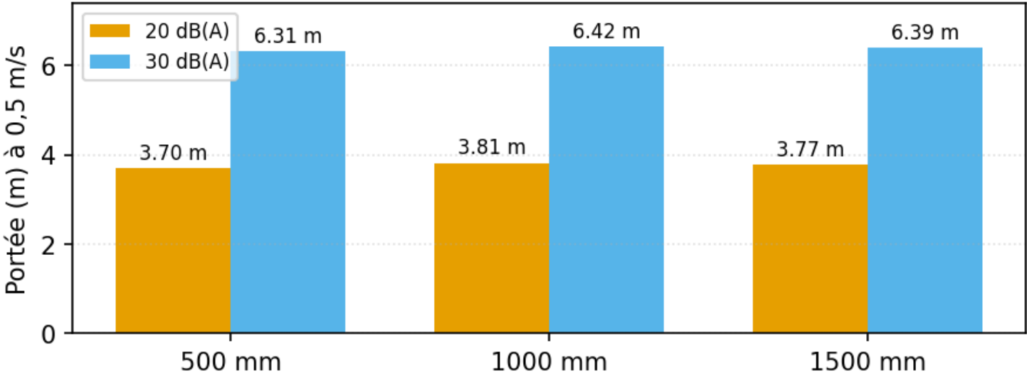
Portée par longueur — C2020 30
