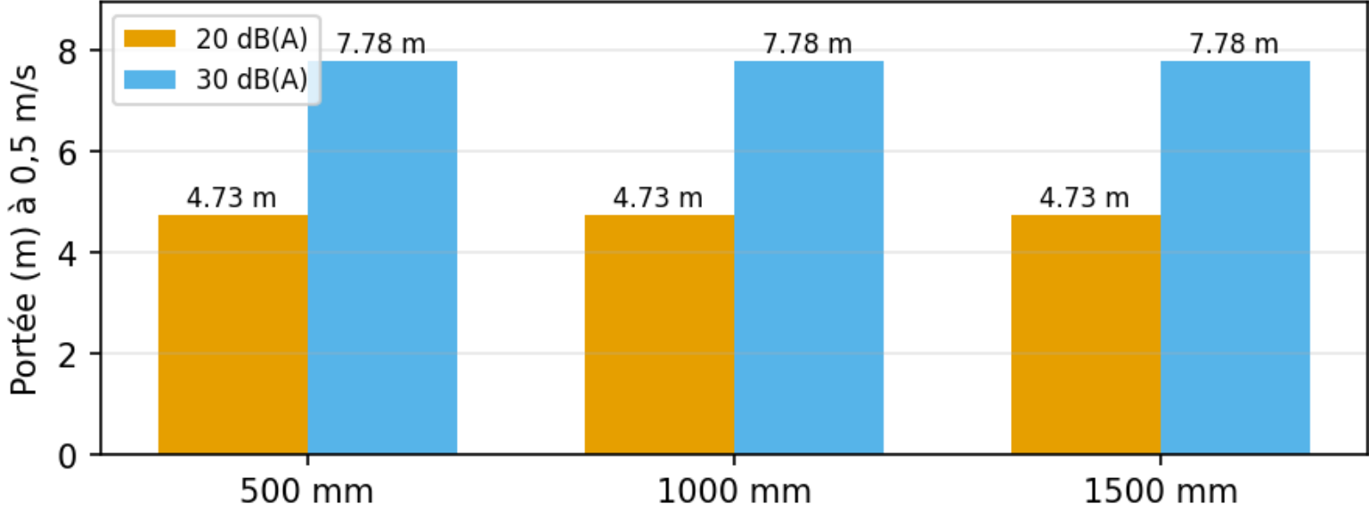
Portée par longueur — C2020 40
