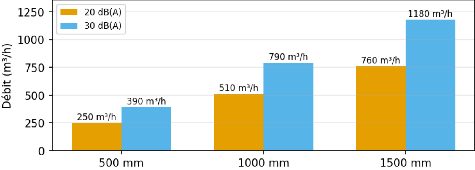
Débit par longueur — C2020 40
