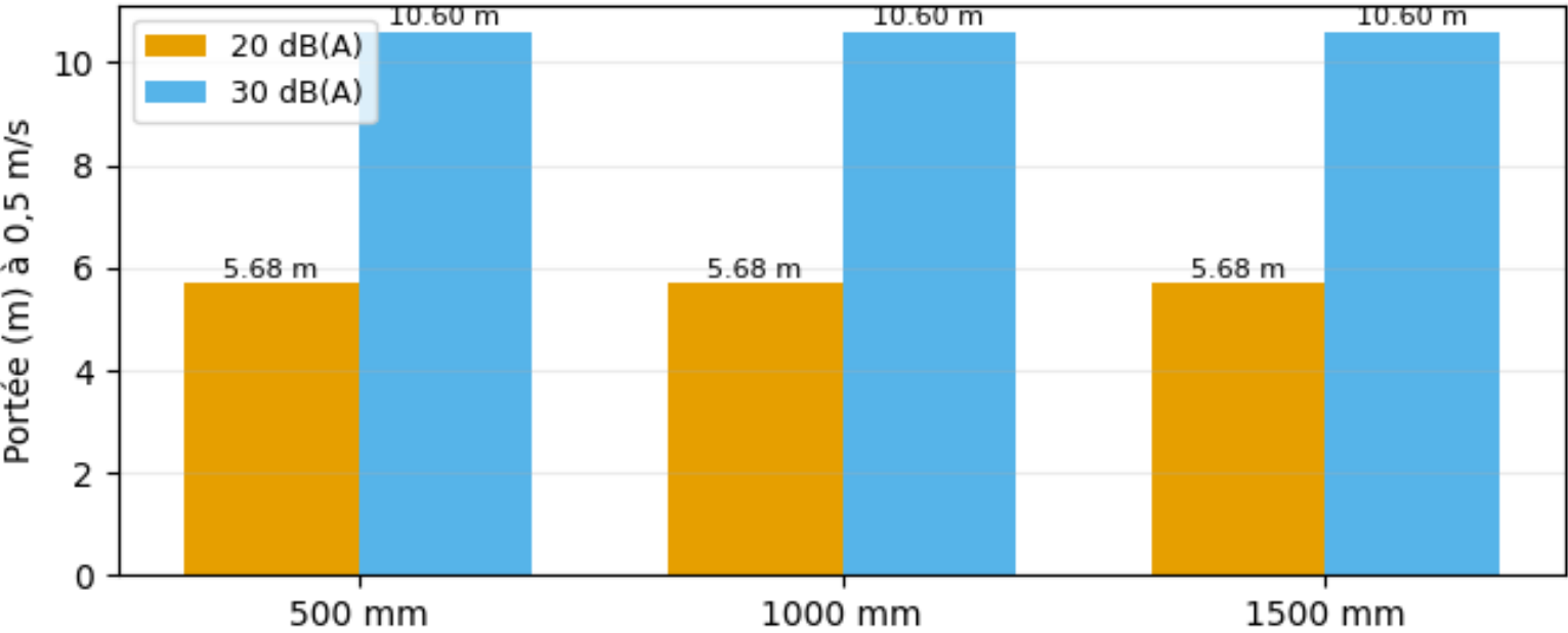
Portée par longueur — C2020 65
