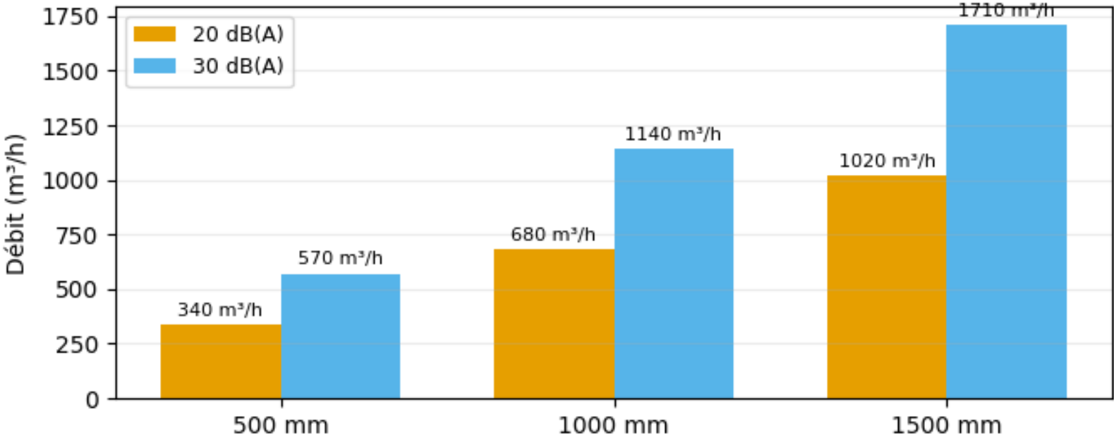
Débit par longueur — C2020 65
