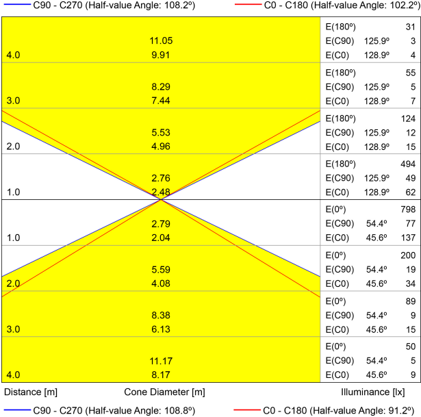
DIAGRAMME CONIQUE
