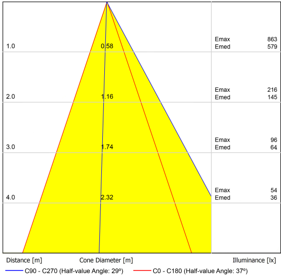
DIAGRAMME CONIQUE
