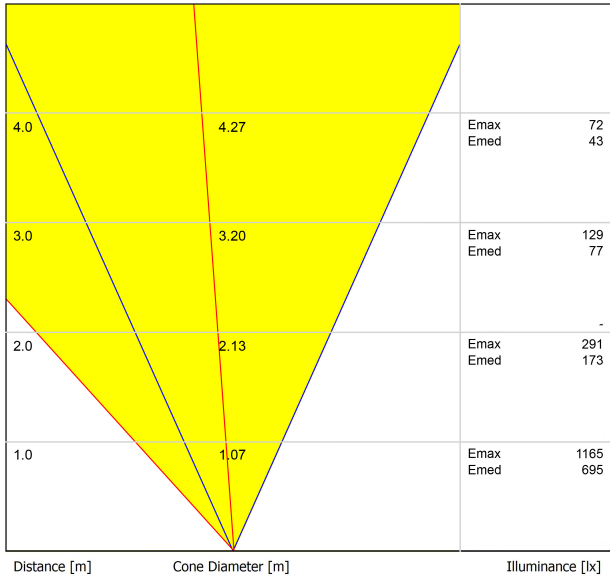
DIAGRAMME CONIQUE
