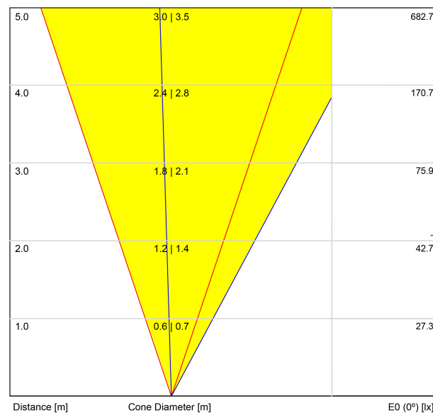
DIAGRAMME CONIQUE
