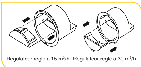
Commutateur 2 vitesses
