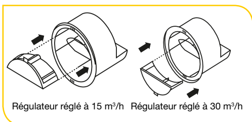
Commutateur 2 vitesses
