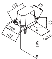
CDVA Contrôleur de débit vitesse d'air à palette IP65.
