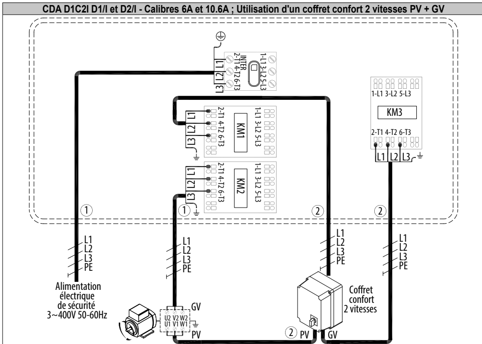
CDA D1C2I D1/I et D2/I - Calibres 6A et 10.6A ; Utilisation d'un coffret confort 2 vitesses PV + GV
