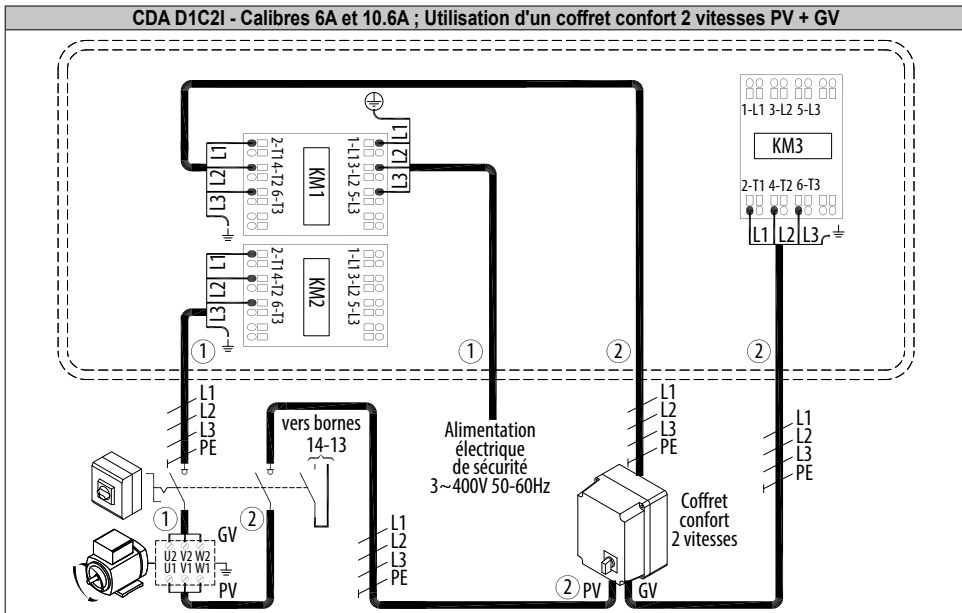
CDA D1C2I D1/I et D2/I - Calibres 6A et 10.6A ; Utilisation d'un coffret confort 2 vitesses PV + GV
