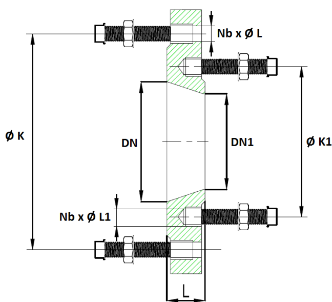
DOUBLE GOUJONNAGE (TYPE DG)
