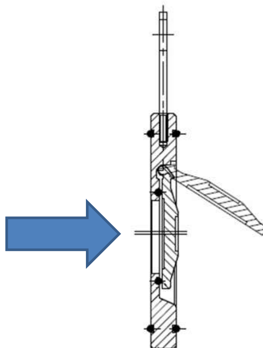
Montage Horizontal
