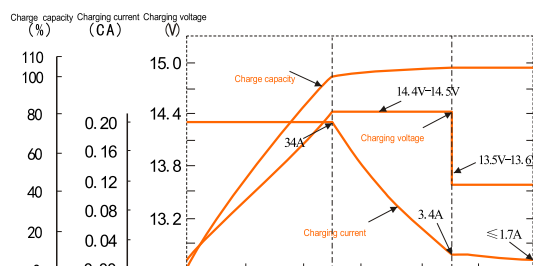
Charge characteristics 77°F (25°C) / Caractéristiques de charge 77°F (25°C)
