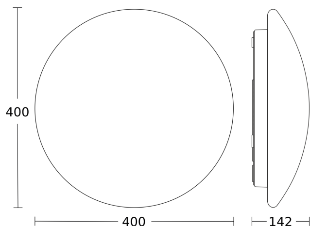
Dessin dimensionnel
