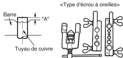
<Type d'écrou à oreilles>
