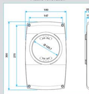
Platine d'adaptation 150/125
