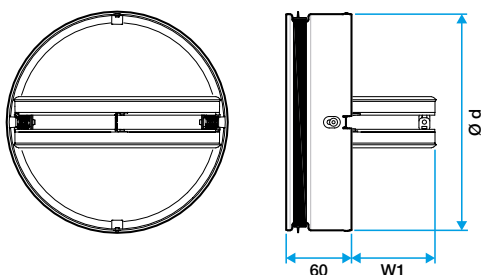
Encombrement (mm)
