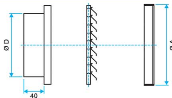
Grille AR 637 de Ø 125 à Ø 315
