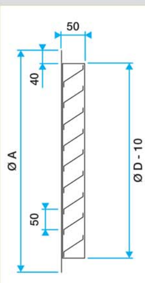
Grille AR 637 de Ø 400 à Ø 630
