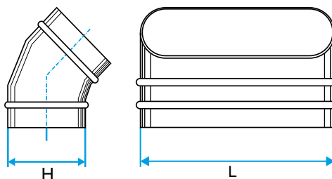
Schéma d'encombrement Coude Vertical Oblong 45°
