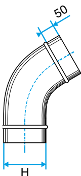
Schéma d'encombrement Coude Vertical Oblong 45°
