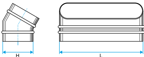
Schéma d'encombrement Coude Vertical Oblong 30°
