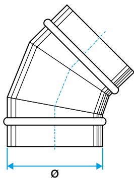
Schéma d'encombrement Coude 45°
