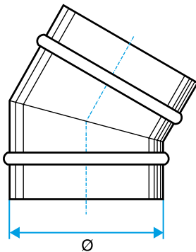
Schéma d'encombrement Coude 30°
