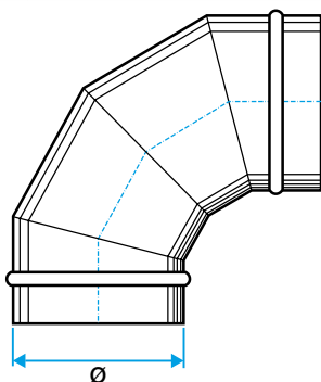
Schéma d'encombrement Coude 90°
