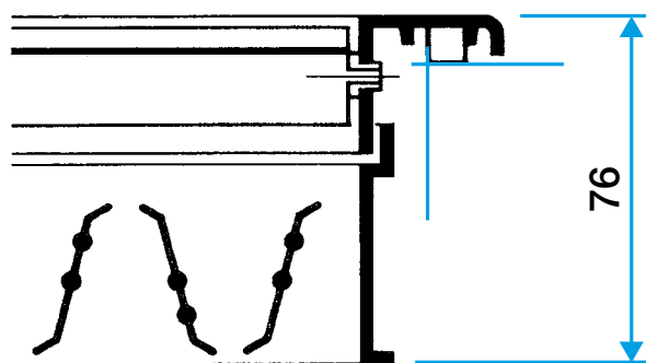
Grille AC 101 avec registre AGB ou SGS monté
