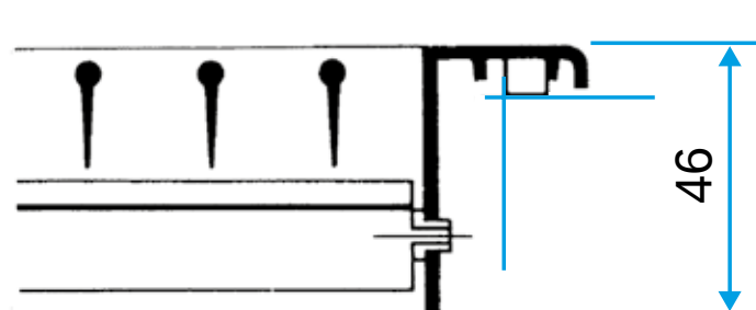
Grille AC 102 D seule
