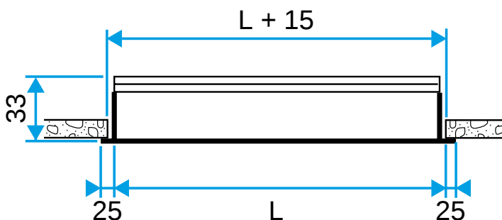
Diffuseur ALD 610 - 620
