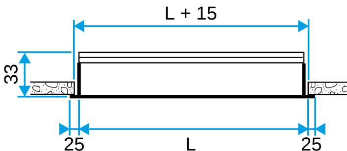
Diffuseur ALD 610 - 620
