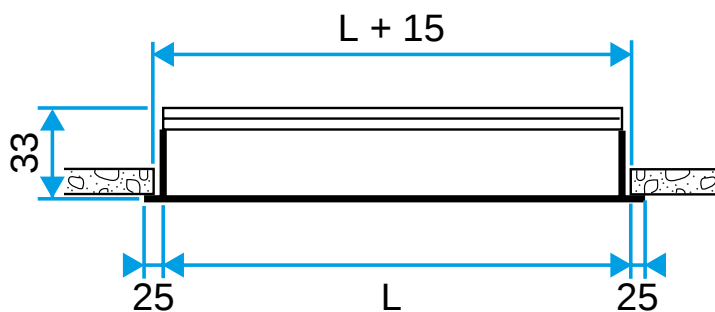
Diffuseur ALD 610 - 620
