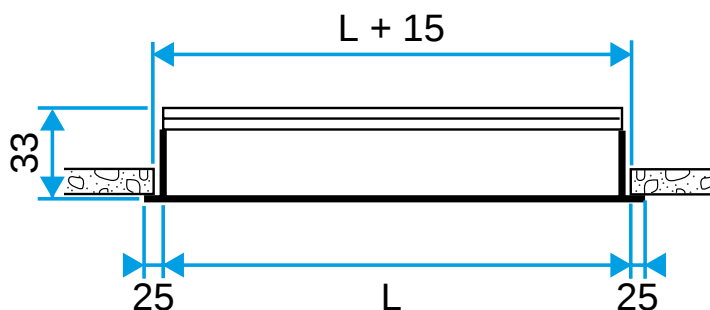
Diffuseur ALD 610 - 620
